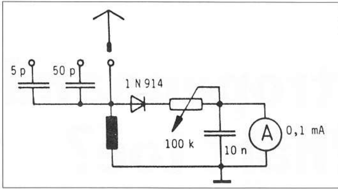
Figuur 1: De veldsterktemeter.
